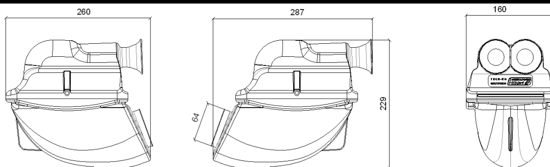
MONTAGEM – OPÇÃO 1
