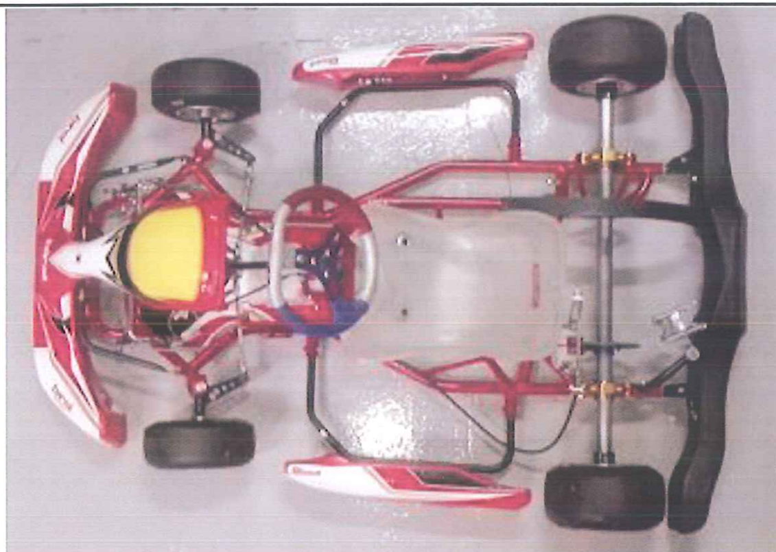
Foto do chassis montado, com pneus
