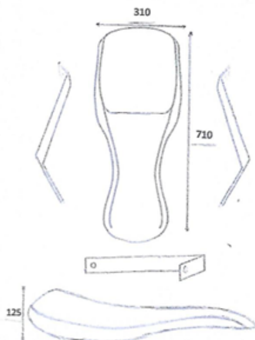
FOTO (conjunto completo com suportes aparentes)
