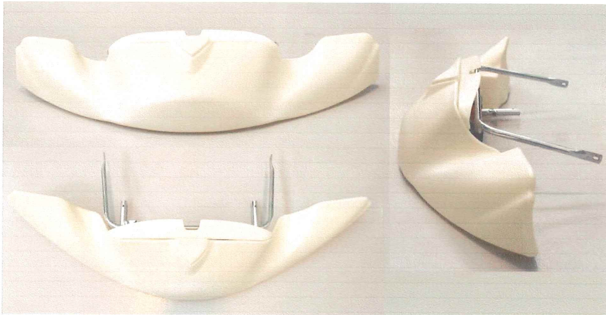
PHOTOS VUE DE DEVANT, DE DESSUS ET DE COTÉ, DU CARENAGE AVANT AVEC SUPPORTS
