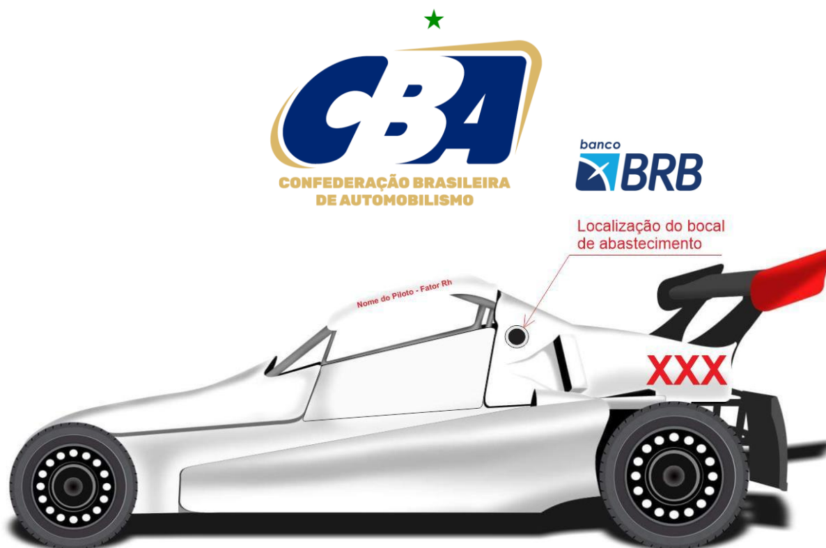
Imagem 12 – posição obrigatória do bocal do tanque de combustível
